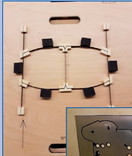
Bandstahlschnitt Schneidlinien in Schichtholz
